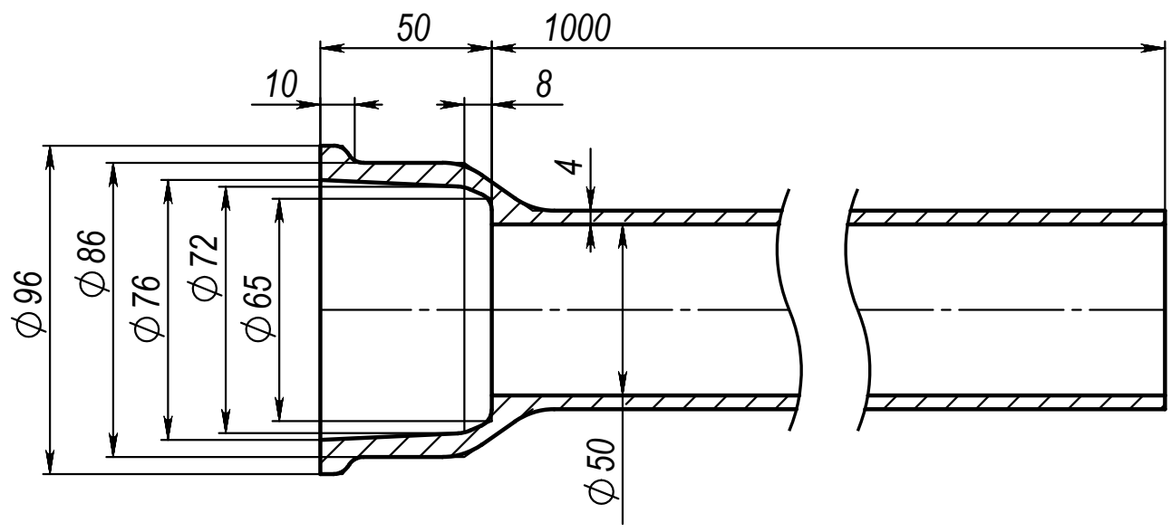
ТЧК-50-1000 ГОСТ 6942-98
