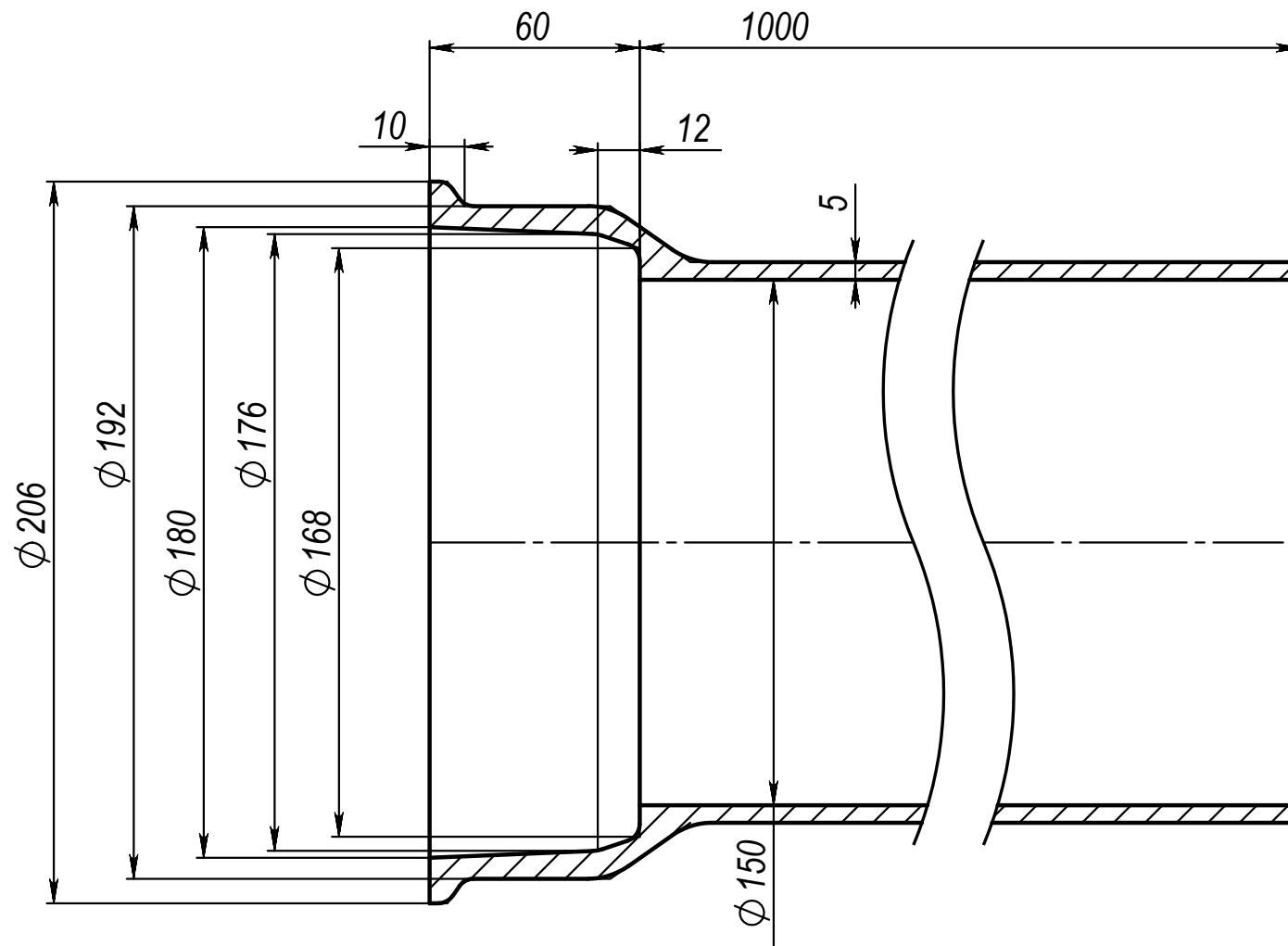
ТЧК-150-1000 ГОСТ 6942-98
